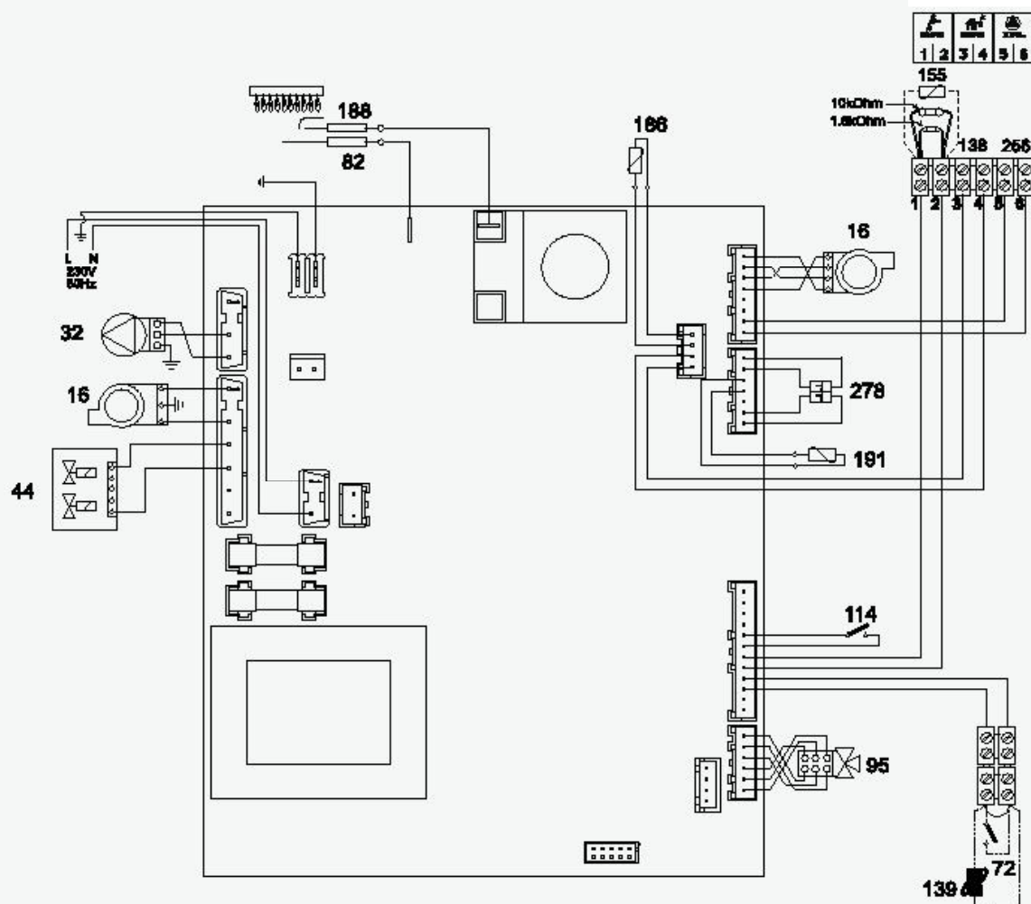
elektrická schéma model
